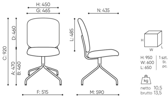
HS 4SO H 4N
