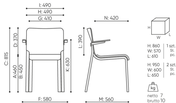
WE 720 2N
