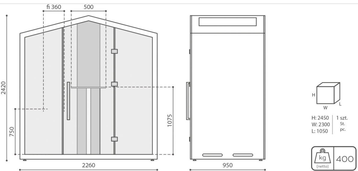
THS 2 TG2 / THSW 2 TG2
